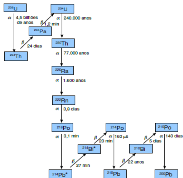
Figura 1 - Esquema de decaimento da série do ^{238}\text{U} . Os símbolos \alpha e \beta ao lado das setas indicam o tipo de decaimento e os tempos mostrados são as meias vidas. O asterisco mostra que o isótopo é emissor gama: Urânio-235, Chumbo-214, Chumbo-211, Bismuto-214, Bismuto-211, Protactínio-231, Tório-227, Tório-232, Frâncio-223, Rádio-223, Radônio-219. Fonte: adaptado de Eisenbud (1973) por Umisedo (2007).
